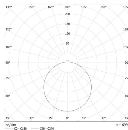
MILEDdo (kat 31220) CORSO LED V2 12-NW / LDC (Polar)
