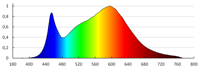
MILEDdo (kat 31220) CORSO LED V2 12-NW / LDC (Polar)
