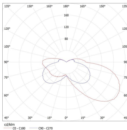
KANLUX S.A. (kat 23108) SABIK LED WW / LDC (Polar)
