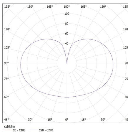
KANLUX S.A. (kat 29612) XLED A60 8W-WW-M / LDC (Polar)
