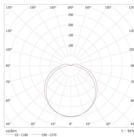
Miledo (kat 31496) TOLU C LED 12W-NW-W / Krzywa rozsyłu światła (biegunowo)
