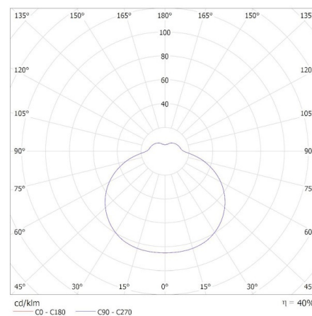
KANLUX S.A. (kat 37325) AMAZI LED 17,5W NW B / Krzywa rozsyłu światła (biegunowo)
