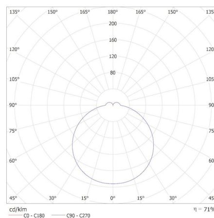
MILED O (kat 31240) DUNO PRO 15W-NW-O / Krzywa rozsyłu światła (biegunowo)
