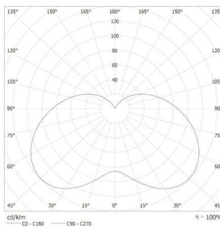
KANLUX S.A. (kat 23439) IDO 6,5W E14-WW / Krzywa rozsyłu światła (biegunowo)
