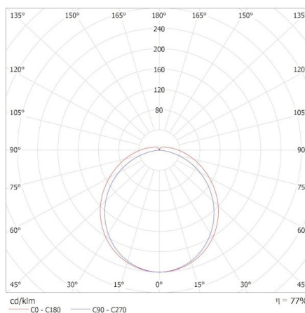
KANLUX S.A. (kat 33893) MEBA LED 40W IP54 NW / Krzywa rozsyłu światła (biegunowo)
