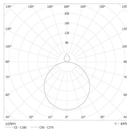
MILED0 (kat 31514) AZPO LED 18,5WCCT-O-W / Krzywa rozsyłu światła (biegunowo)
