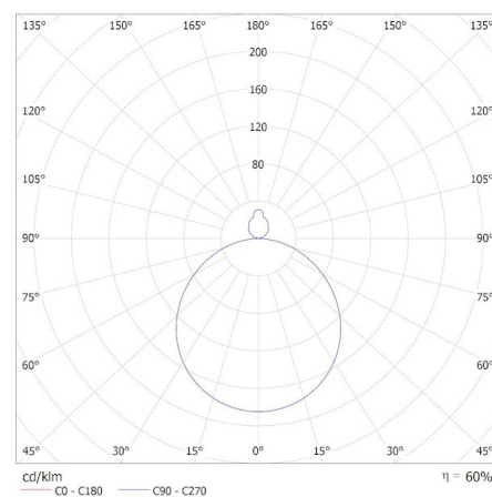
MILED O (kat 31515) AZPO LED 18,5WCCT-O-B / Krzywa rozsyłu światła (biegunowo)
