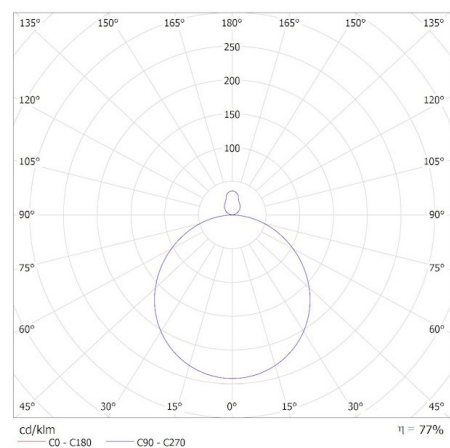
MILED0 (kat 31516) AZPO LED 22WCCT-O-W / Krzywa rozsyłu światła (biegunowo)
