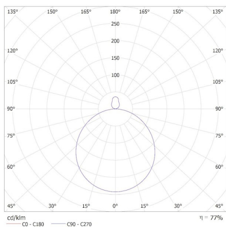
MILED0 (kat 31517) AZPO LED 22WCCT-O-B / Krzywa rozsyłu światła (biegunowo)
