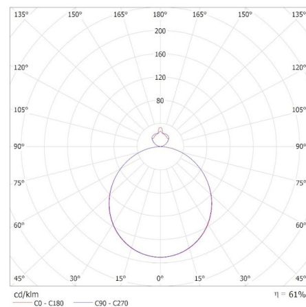
MILED O (kat 31530) AZPO LED 12,3WCCT-L-W / Krzywa rozsyłu światła (biegunowo)
