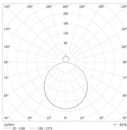
MILED O (kat 31531) AZPO LED 12,3WCCT-L-B / Krzywa rozsyłu światła (biegunowo)
