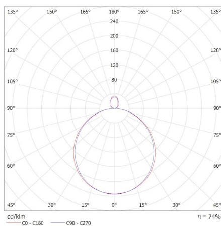
MILED0 (kat 31535) AZPO LED 22WCCT-L-B / Krzywa rozsyłu światła (biegunowo)
