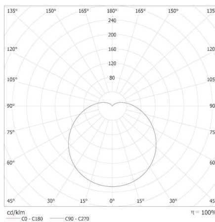
KANLUX S.A. (kat 36689) IQ-LED G45E14 3,4W-NW / Krzywa rozsyłu światła (biegunowo)
