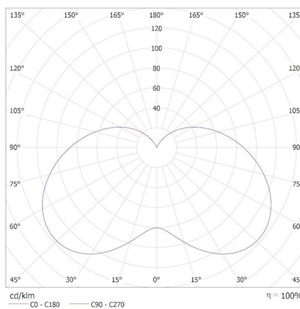
KANLUX S.A. (kat 36686) IQ-LED C35E14 5,9W-NW / Krzywa rozsyłu światła (biegunowo)
