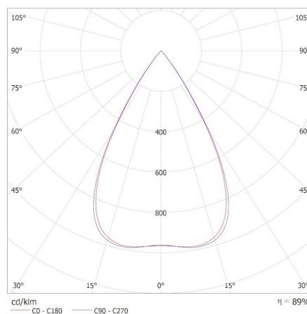
KANLUX S.A. (kat 37028) HR-MH-WW-W-PT / Krzywa rozsyłu światła (biegunowo)
