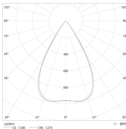
KANLUX S.A. (kat 37027) HR-MM-WW-W-PT / Krzywa rozsyłu światła (biegunowo)
