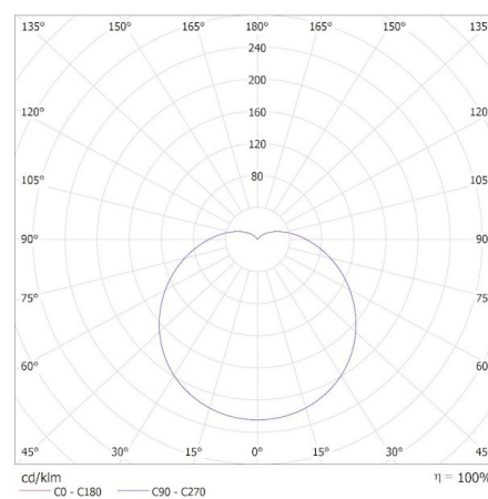
KANLUX S.A. (kat 36690) IQ-LED G45E14 3,4W-CW / Krzywa rozsyłu światła (biegunowo)
