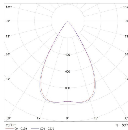
KANLUX S.A. (kat 36944) HR-MH-WW-W-NT / Krzywa rozsyłu światła (biegunowo)
