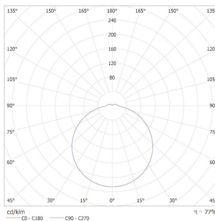
KANLUX S.A. (kat 37293) IPER LED 35W-NW-O / Krzywa rozsyłu światła (biegunowo)
