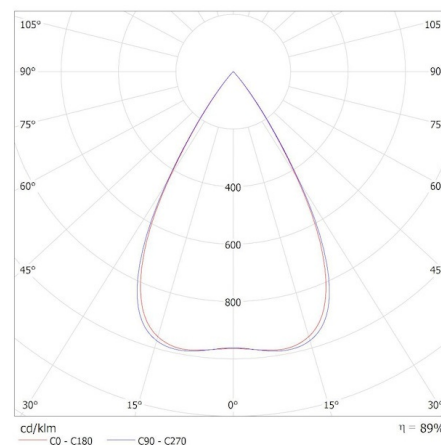
KANLUX S.A. (kat 37059) HR-MM-NW-W-PT / Krzywa rozsyłu światła (biegunowo)
