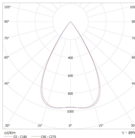
KANLUX S.A. (kat 37042) HR-ML-WN-W-PT / Krzywa rozsyłu światła (biegunowo)
