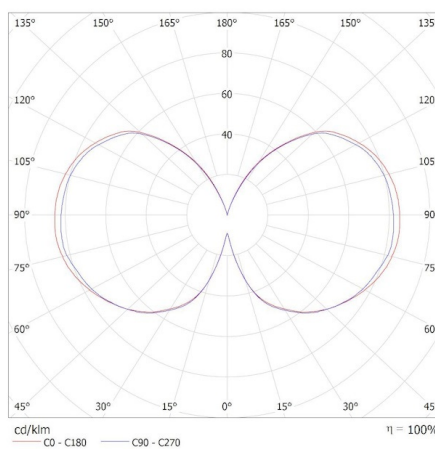
KANLUX S.A. (kat 37241) XLEDIM A60 E27 11W-NW / Krzywa rozsyłu światła (biegunowo)
