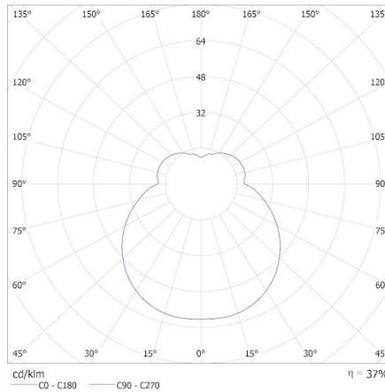
KANLUX S.A. (kat 38034) PLAVE LED CCT+RGB - nw / Krzywa rozsyłu światła (biegunowo)
