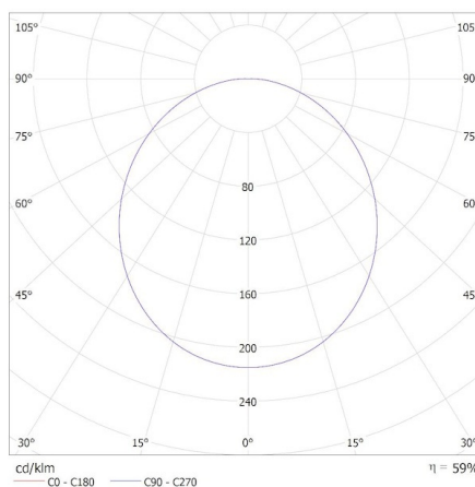
KANLUX S.A. (kat 38790) BENO 12-18W CCT-O-SEG 12W / Krzywa rozsyłu światła (biegunowo)
