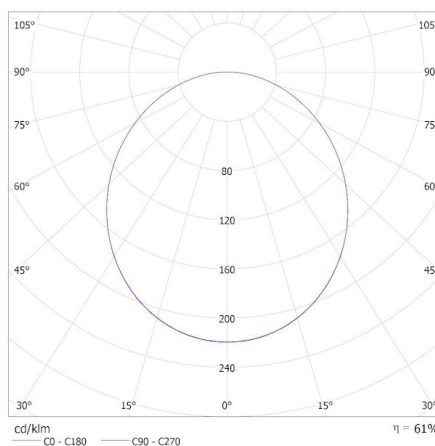
KANLUX S.A. (kat 38788) BENO 12-18W CCT-L-SEG 12W / Krzywa rozsyłu światła (biegunowo)
