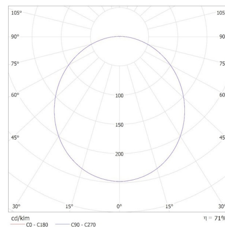
KANLUX S.A. (kat 38781) BENO 24-30W CCT-L-SEW 24W / Krzywa rozsyłu światła (biegunowo)
