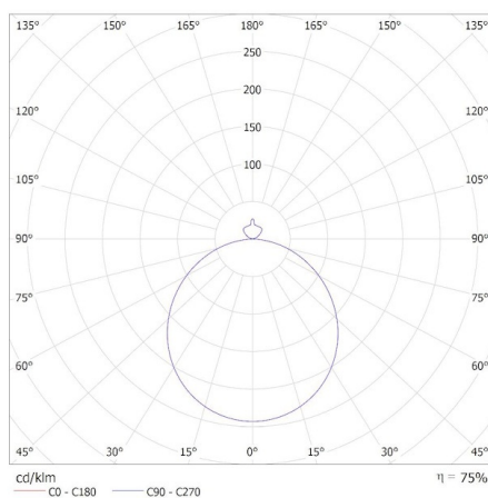
MILEDO (kat 31512) AZPO LED 11,8WCCT-O-W / Krzywa rozsyłu światła (biegunowo)
