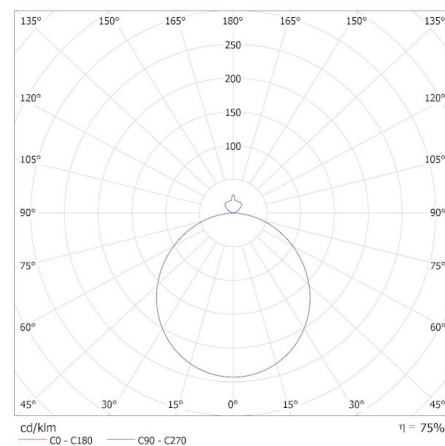
MILED (kat 31513) AZPO LED 11,8WCCT-O-B / Krzywa rozsyłu światła (biegunowo)
