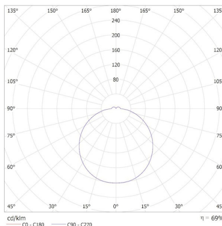
MILED0 (kat 31491) TURA LED 24W-NW-O-B / Krzywa rozsyłu światła (biegunowo)
