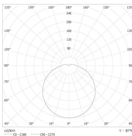
Miledo (kat 31497) TOLU O LED 9W-NW-W / Krzywa rozsyłu światła (biegunowo)
