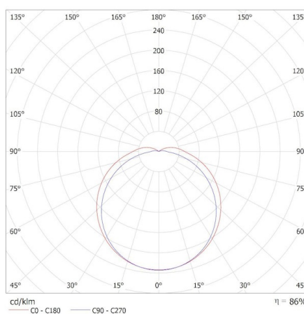
Miledo (kat 31495) TOLU C LED 6W-NW-W / Krzywa rozsyłu światła (biegunowo)
