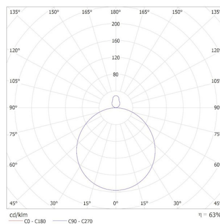
MILED O (kat 31505) AZPO LED 22W-NW-O-B / Krzywa rozsyłu światła (biegunowo)
