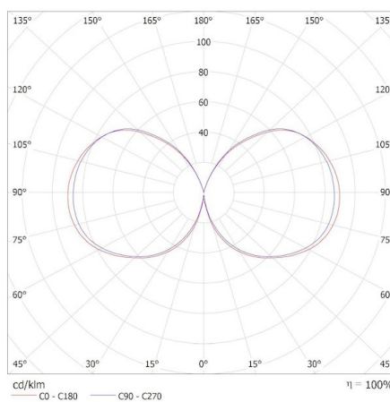
KANLUX S.A. (kat 38416) XLED C35E14 7W-WW / Krzywa rozsyłu światła (biegunowo)
