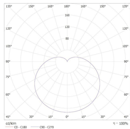
KANLUX S.A. (kat 26767) BILO 6,5W E14-WW / Krzywa rozsyłu światła (biegunowo)
