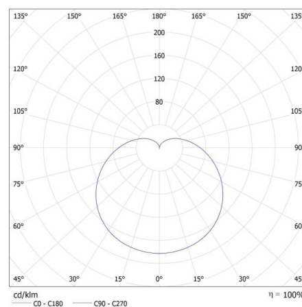
MILED O (kat 31205) A60 N 9,5W E27-NW / LDC (Polar)
