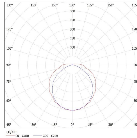
KANLUX S.A. (kat 26961) MEBA 4LED 2X120 PS + GLASSv4 / LDC (Polar)
