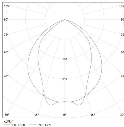
KANLUX S.A. (kat 22671) NOTUS 4LED 418 NT + GLASSv4 / LDC (Polar)
