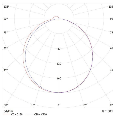
KANLUX S.A. (kat 26683) ASTEN IP44 8W-NW-B / LDC (Polar)
