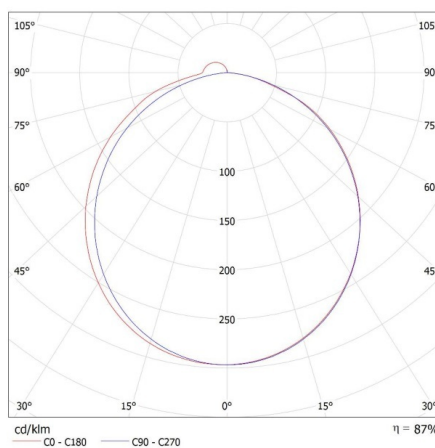
KANLUX S.A. (kat 26688) ASTEN IP44 15W-NW-W / LDC (Polar)
