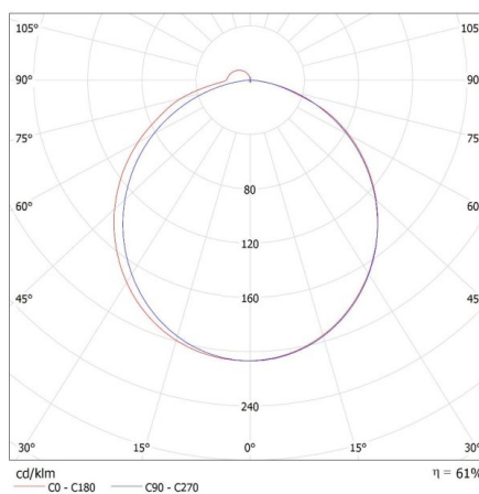
KANLUX S.A. (kat 26685) ASTEN IP44 15W-NW-B / LDC (Polar)
