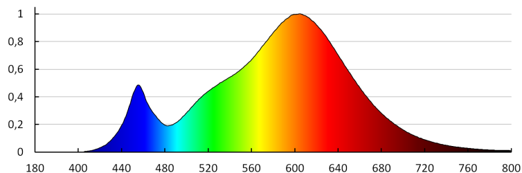
MILED O (kat 31202) A60 N 8W E27-WW / LDC (Polar)
