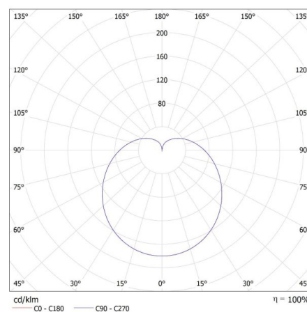
MILED O (kat 31202) A60 N 8W E27-WW / LDC (Polar)
